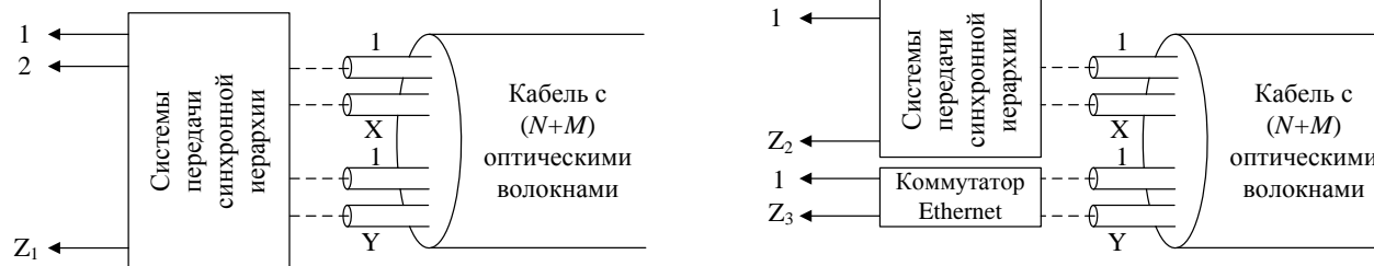
а) Интегральное решение (создание интерфейсов E1)
